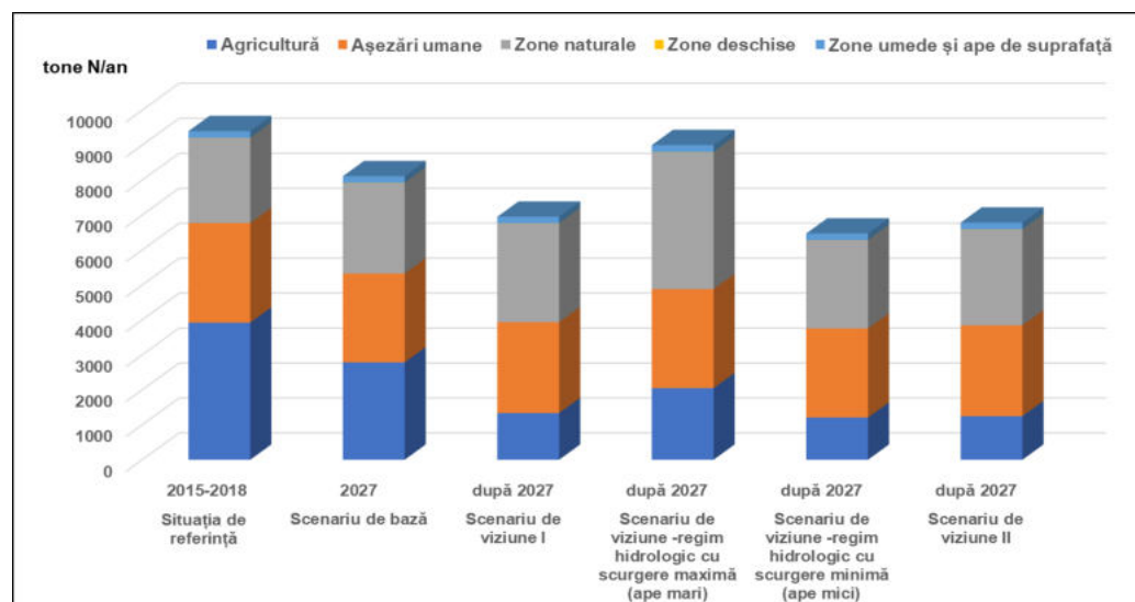
Figura 3.18. Evoluția emisiilor de azot total (pe surse) în funcție de scenarii (exprimate în tone N pe an)
