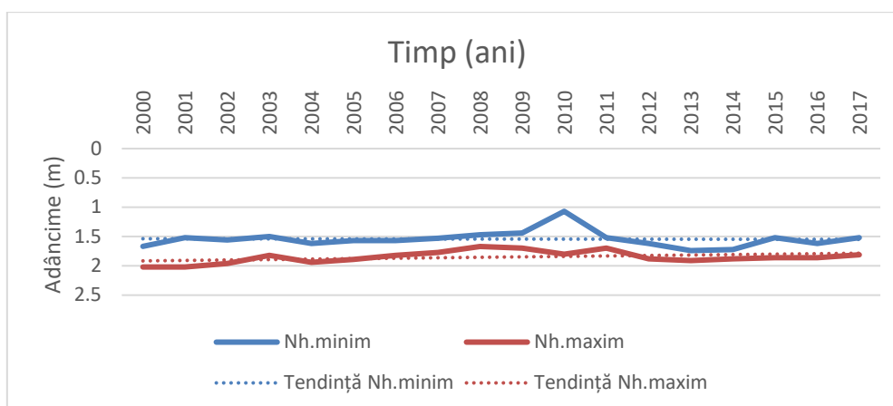
Figura 4.14. Variația adâncimii minime și maxime anuală a nivelului hidrostatic (m) măsurată față de cota terenului, în perioada 2000-2017, în forajul F7 Ionaseni situat în nord-vestul sitului ROSCI0391, aparținând corpului de apă subterană freatic ROSI03
