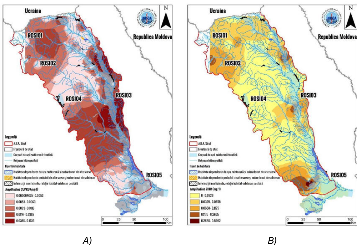
Figura 4.26. Variația diferenței dintre valoarea maximă și minimă a parametrilor chimici cupru (A) și zinc (B) în arealul habitatelor dependente de subterană
