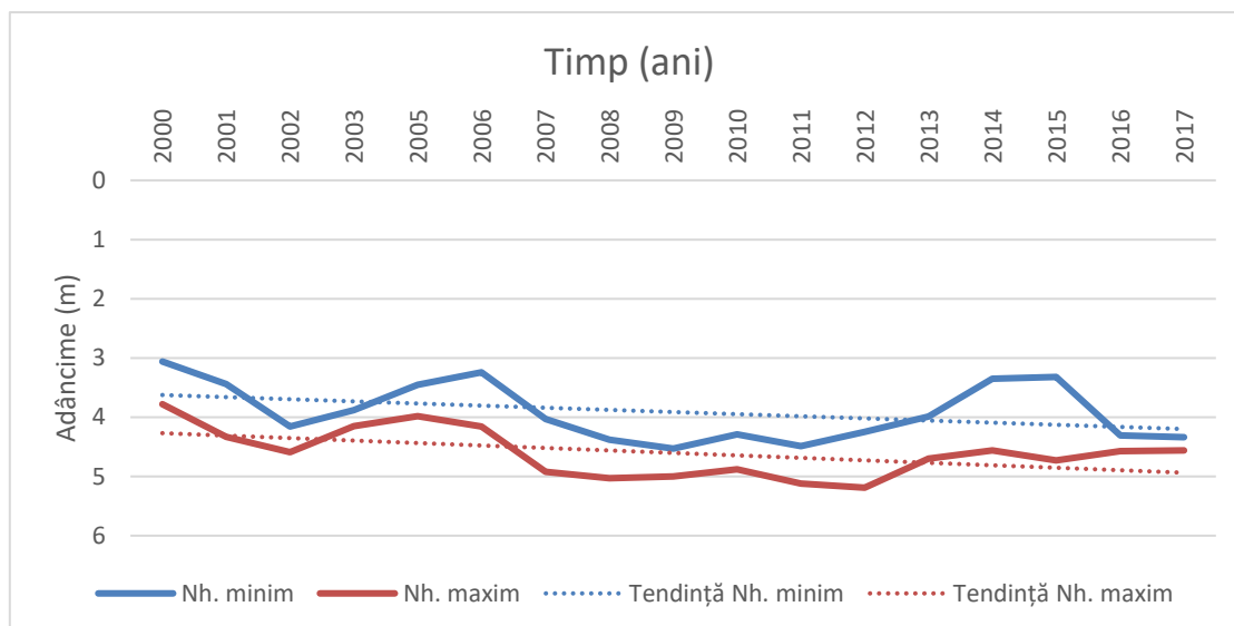
Figura 4.22. Variația adâncimii minime și maxime anuale a nivelului hidrostatic (m) măsurată față de cota terenului, în perioada 2000-2017, în forajul F26 Cilibia Nord situat în centrul sitului ROSCI0103, aparținând corpului de apă subterană freatic ROSI05
