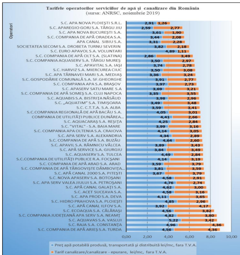
Figura 8.3. Tarife operatori servicii de apă și canalizare
