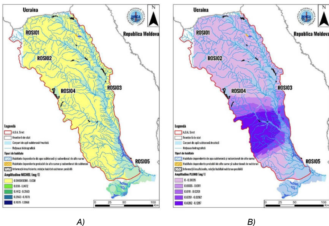
Figura 4.25. Variația diferenței dintre valoarea maximă și minimă a parametrilor chimici nichel (A) și plumb (B) în arealul habitatelor dependente de subterană
