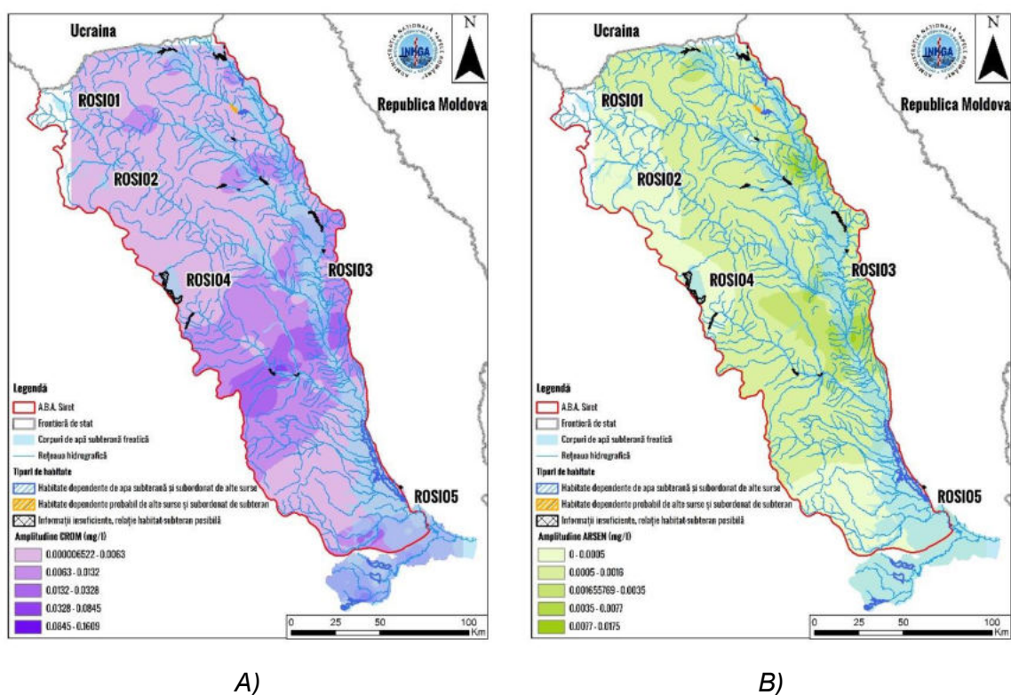
Figura 4.27. Variația diferenței dintre valoarea maximă și minimă a parametrilor chimici crom (A) și arsen (B) în arealul habitatelor dependente de subterană
