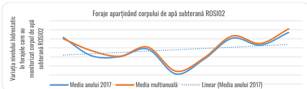
Figura 6.29. Evoluția mediei nivelurilor hidrostatice multianuale și a mediei anuale în anul 2017 pentru corpul de apă subterană ROSI02
