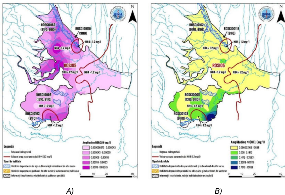
Figura 4.30. Variația conținutului de amoniu și mercur (A), nichel (B) în arealul habitatelor dependente de corpul de apă subterană ROSI05
