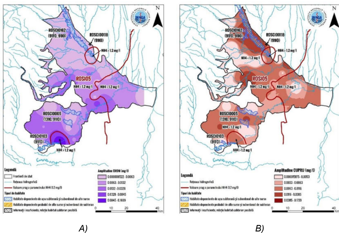
Figura 4.29. Variația conținutului de amoniu și crom (A), cupru (B) în arealul habitatelor dependente de corpul de apă subterană ROSI05
