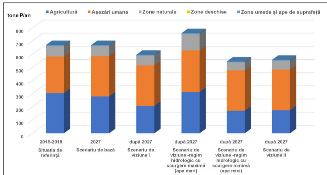
Figura 3.19. Evoluția emisiilor de fosfor total (pe surse) în funcție de scenarii (exprimate în tone P pe an)
